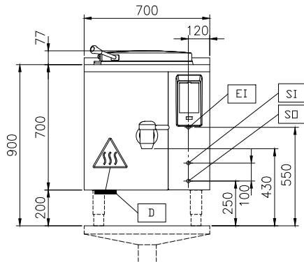
Front aanzicht
